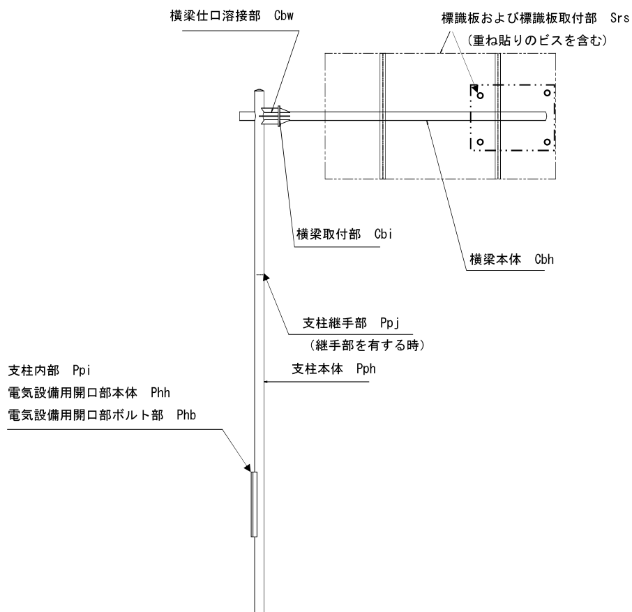
図一 4 標識：逆 L 型
