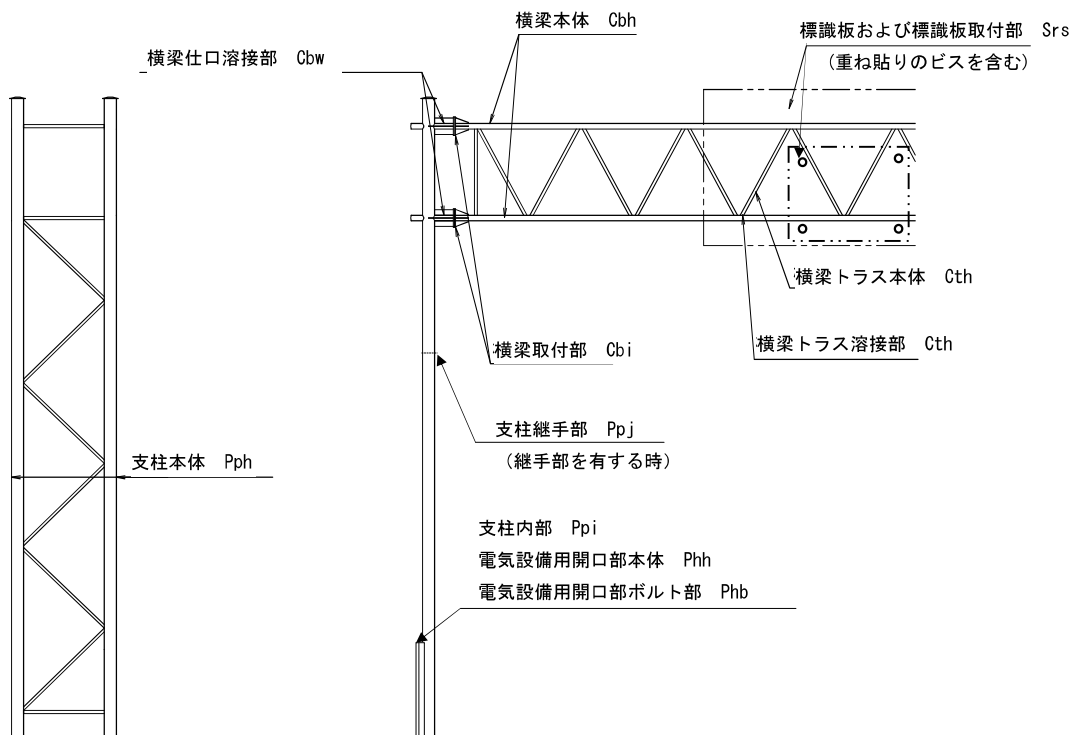
図一 6 標識：トラス門柱型
