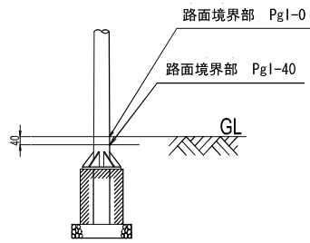
(基礎形式①)
