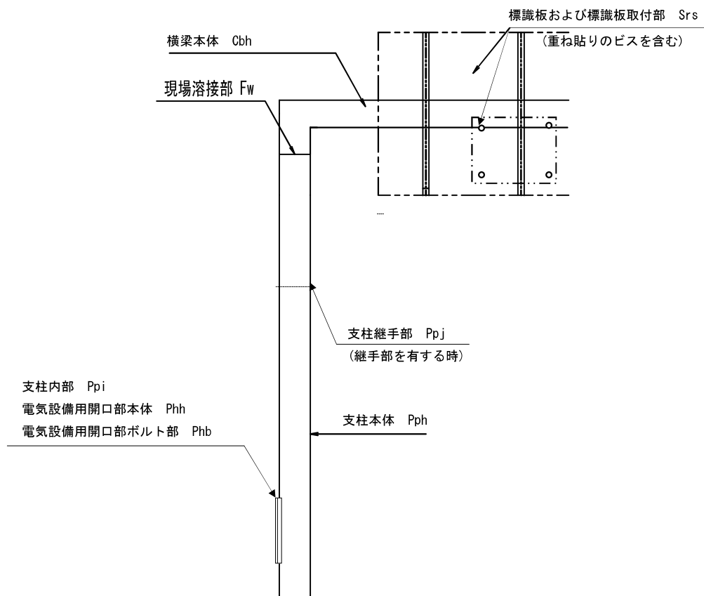
図－７ 標識：アーチ門柱型
