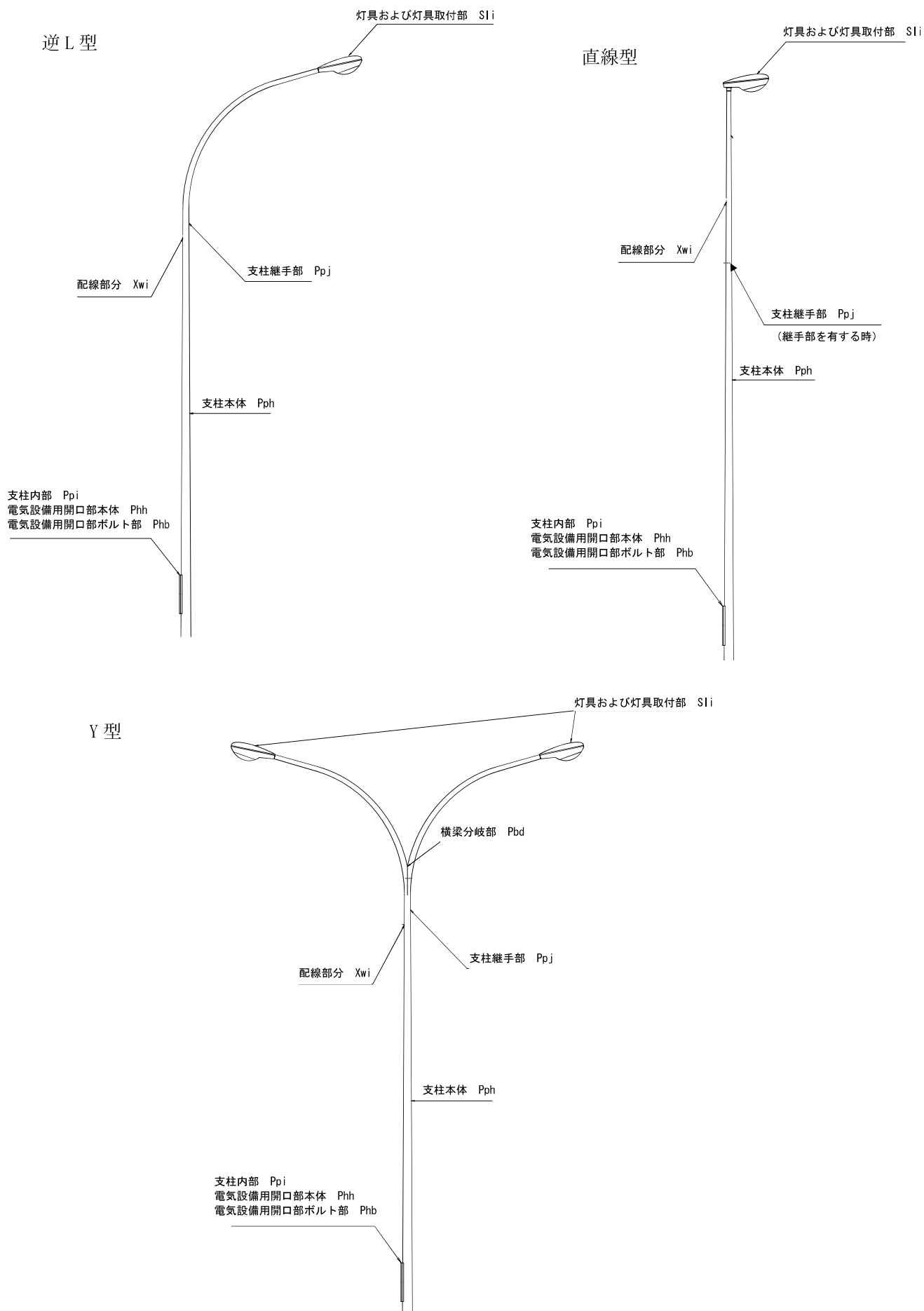
図-9 主な点検箇所（ポール照明方式）
