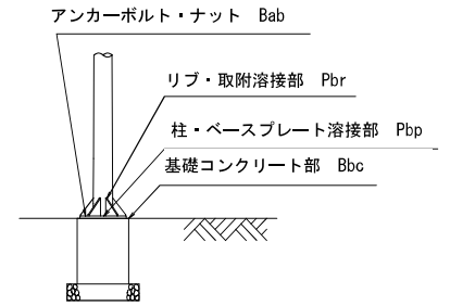
(基礎形式③)
