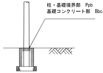
(基礎形式②)
