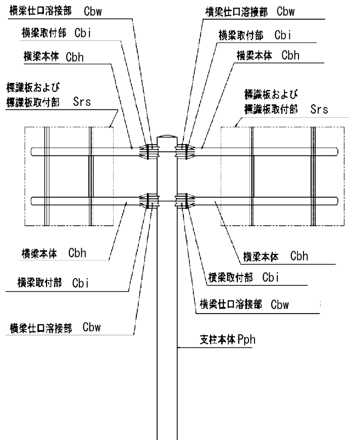
図一 5 標識：T 型
