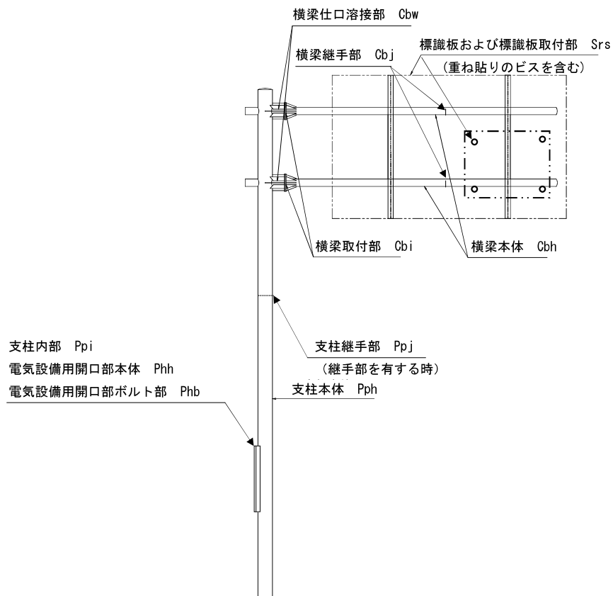
図一 3 標識：F 型
