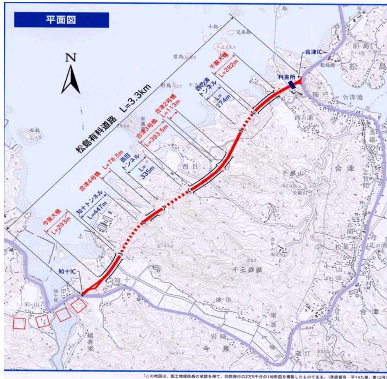
舗装構造調査(FWD)委託 位置図
