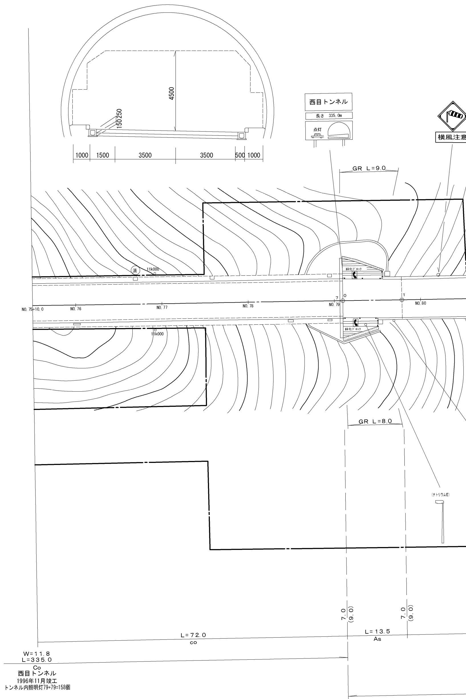
西目トンネル断面図
