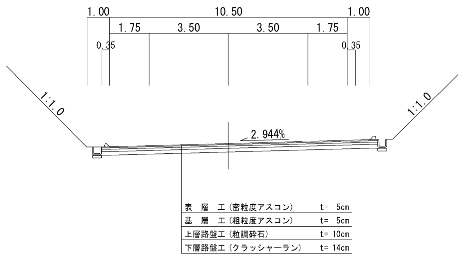
標準断面図 (切土部)
