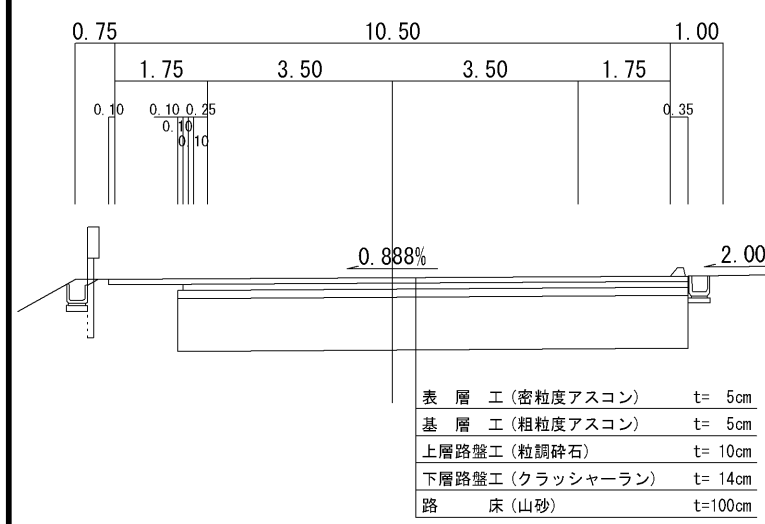
標準断面図
