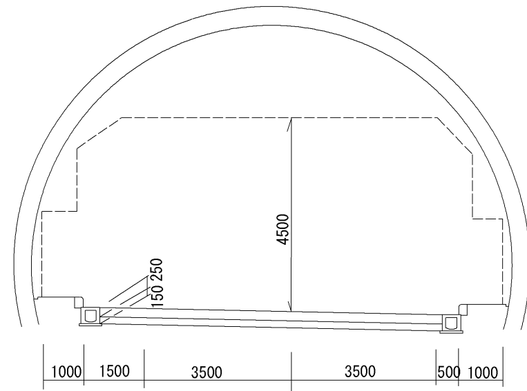
西の浦トンネル断面図
