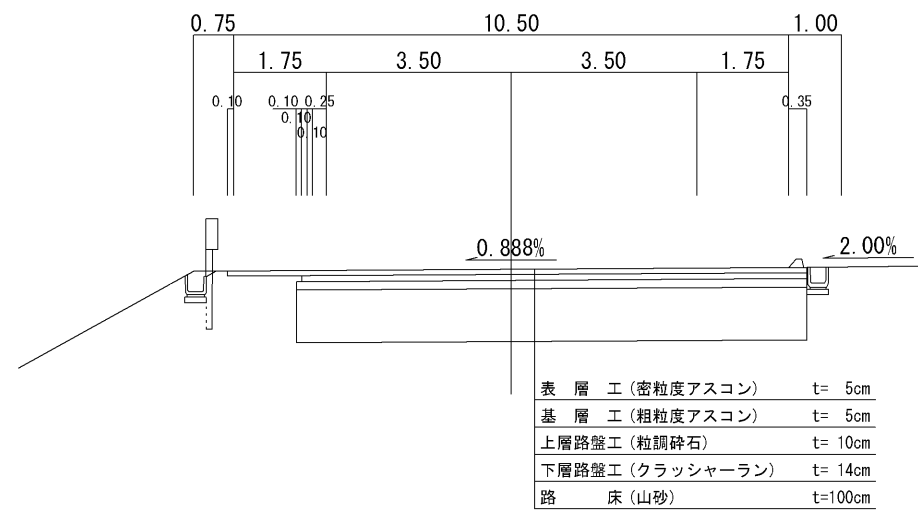
標準断面図 (盛土部)
