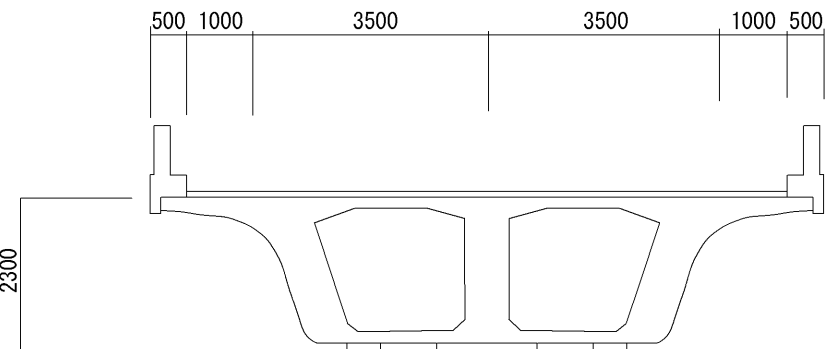
合津3号橋断面図
